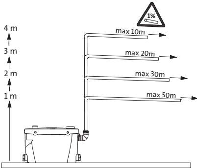
9. ábra Csővezeték
